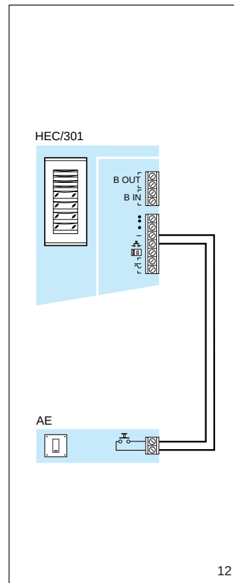
Fig.12-Schema di collegamento del pulsante ausiliario apriporta (AE).
