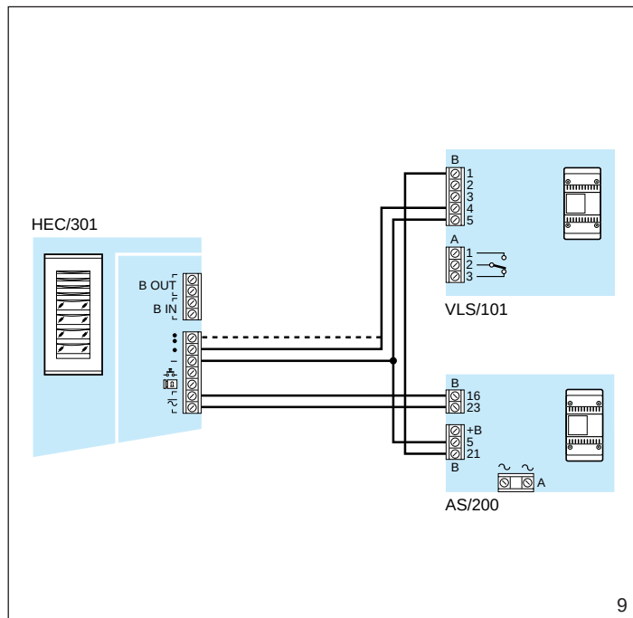
Fig.8-9 Esempio di collegamento uscita ausiliaria Aux 1 o Aux 2 con l'unità relè VLS/101. Alimentazione mediante VAS/100 e AS/200.
