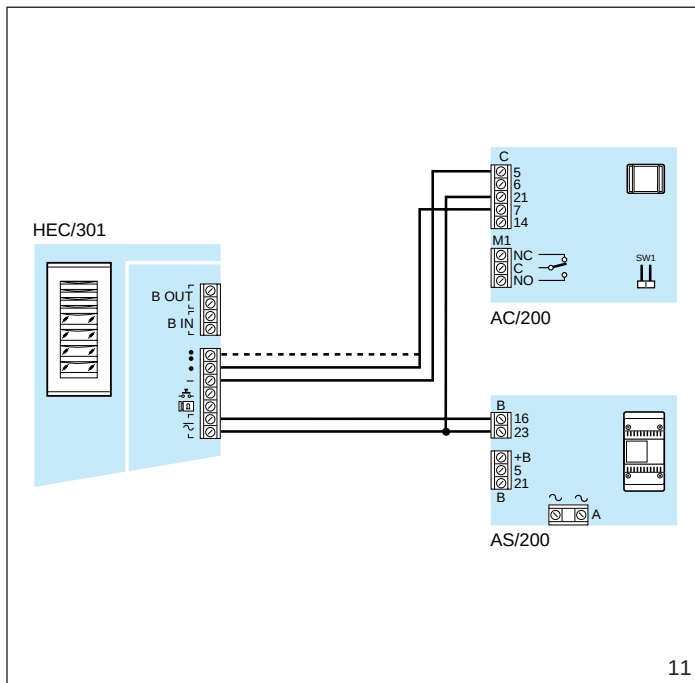
Fig.10-11 Esemplio di collegamento uscita ausiliaria Aux 1 o Aux 2 con l'unità relè AC/200. Alimentazione mediante VAS/100 e AS/200.
