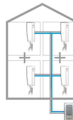
A) Exemple d'extension à l'intérieur d'une habitation uni-familiale
