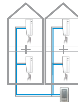
B) Exemple d'extension pour les installations d'habitations bi-familiales
