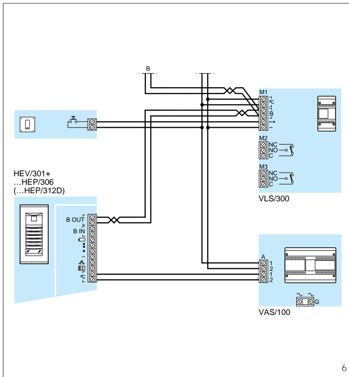
Fig. 5 - Esempio di collegamento dell'unità relè VLS/300 in modalità di funzionamento Master in un impianto sistema 300.
