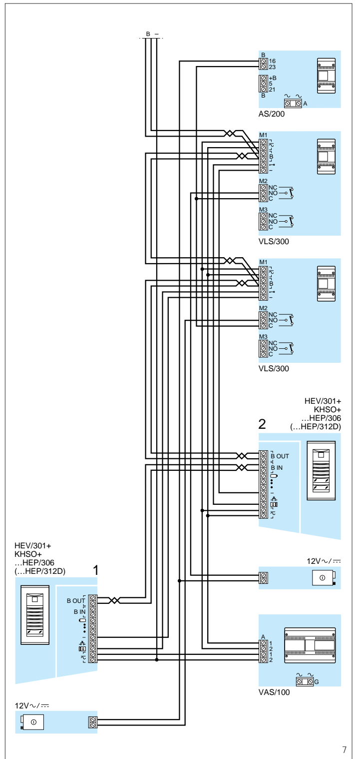
Fig. 6 - Ejemplo de conexión de la unidad relé VLS/300 en modalidad de funcionamiento Master en una instalación sistema X2.
