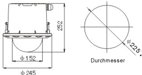
Abmessungen
