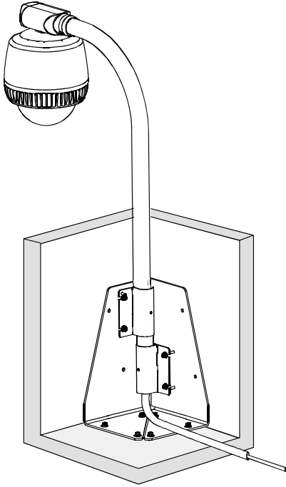
RHOPN pendant mount
